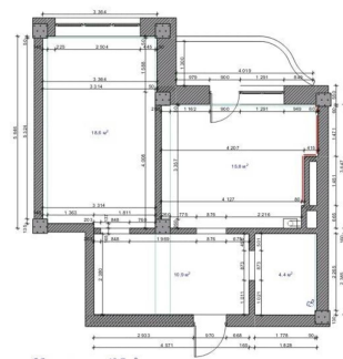
ОБМЕРНЫЙ ПЛАН
